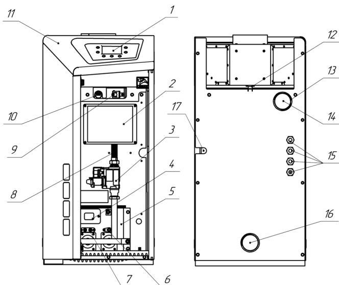
Рис. 1. Конструкция котла.
